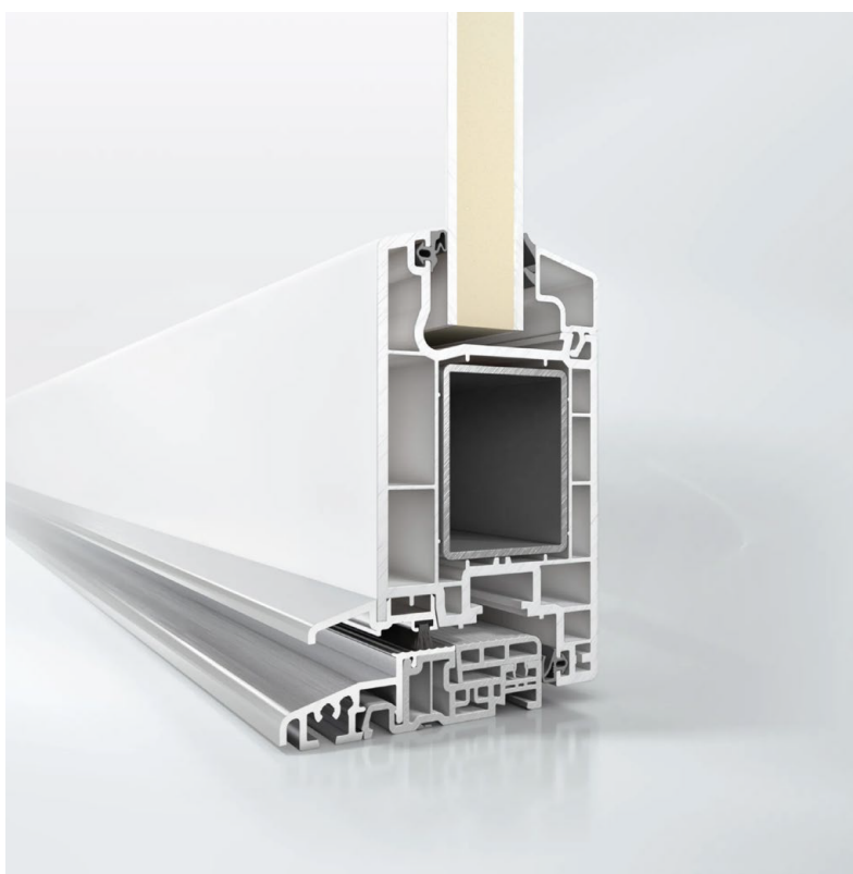
Dettaglio soglia per porta senza barriere
